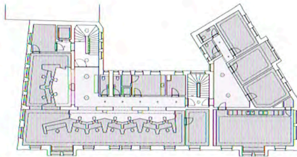
heutiger Zustand 2011, 1. Obergeschoss
