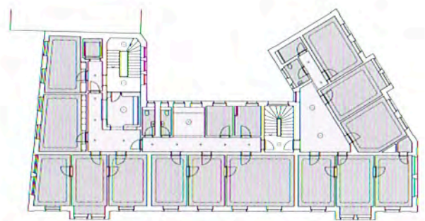
heutiger Zustand 2011, 2. Obergeschoss
