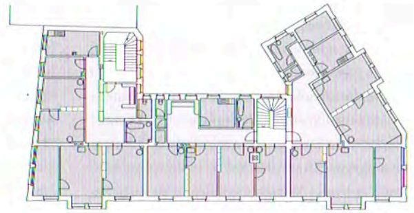
Originalzustand 1910, 2. Obergeschoss
