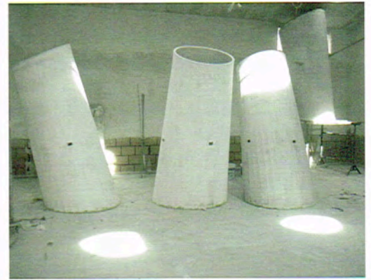
^ Dach und Deckenuntersicht der Reformierten Kirche in Dornach sind unterschiedlich gefaltet – die Zylinder der Oberlichter entsprechend unterschiedlich lang.
